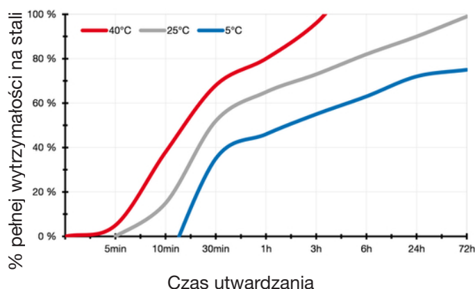
Szybkość reakcji w różnych temperaturach
