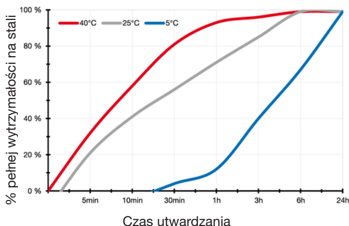
Szybkość reakcji w różnych temperaturach
