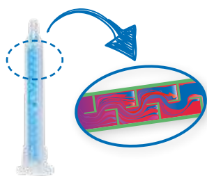
QUADRO-zmiešavacia dýza A
