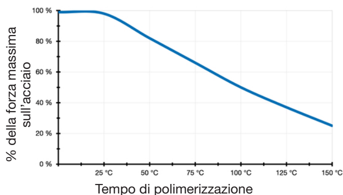
Velocità di reazione a diverse temperature
