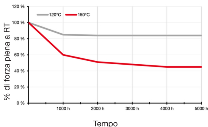
Invecchiamento termico
