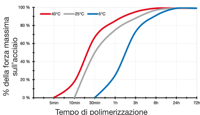
Velocità di reazione di vari materiali
