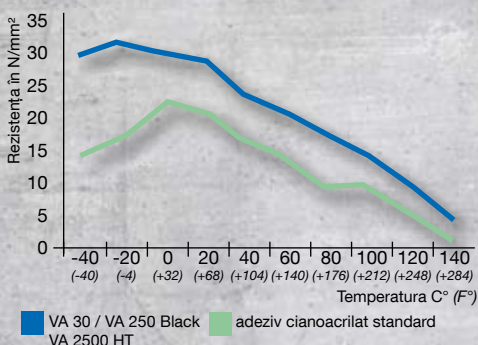
Graficul rezistenței lipirii în funcție de temperatură
