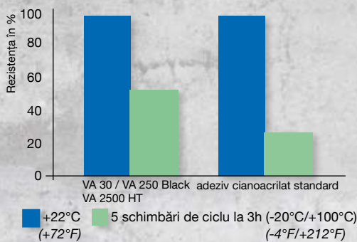
Rezistența în climat umed
