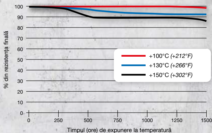
Rezistența la temperatură a WEICONLOCK pe termen lung la temperaturi înalte
