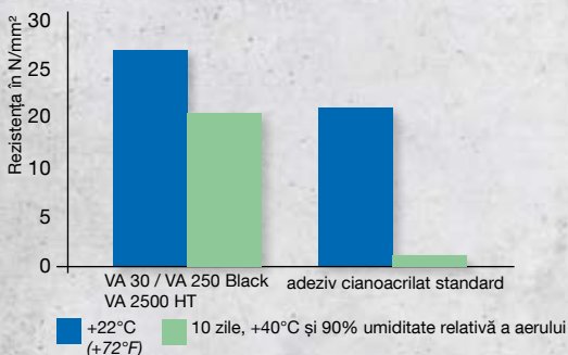
Îmbătrânirea pe termen scurt la +140°C
