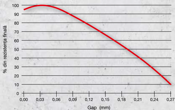
Rezistența WEICONLOCK În funcție de mărimea interstițiului
