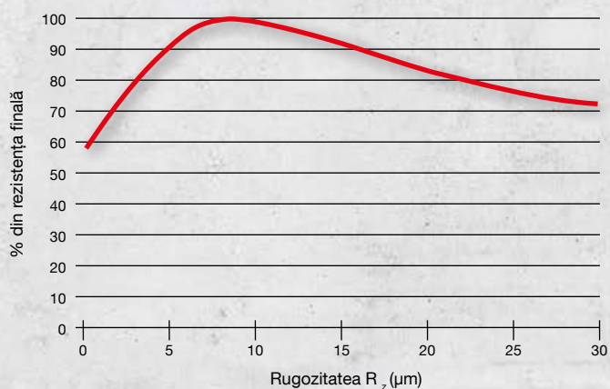
Rezistența WEICONLOCK În funcție de rugozitate
