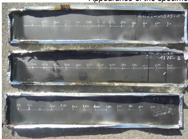
Aussehen der Proben nach dem Cone Versuch Appearance of the specimen after the cone test
