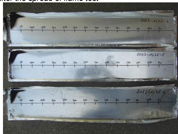
Aussehen der Proben nach dem Spread of Flame Versuch Appearance of the specimen after the spread of flame test
