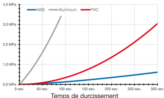
Vitesse de réaction de divers matériaux
