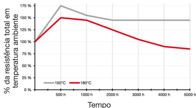
Envelhecimento térmico
