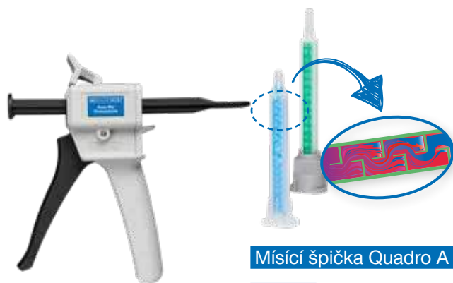
Dávkovací pistole D50
