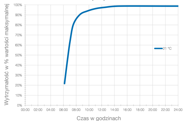
Wzrost wytrzymałości
