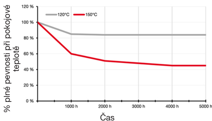
Teplotní stárnutí
